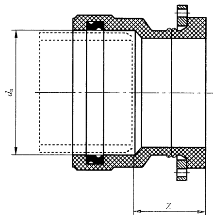
图 A.5 法兰和承口接头示意图
