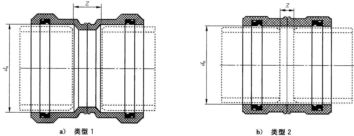
图 A.3 双承口套筒示意图
