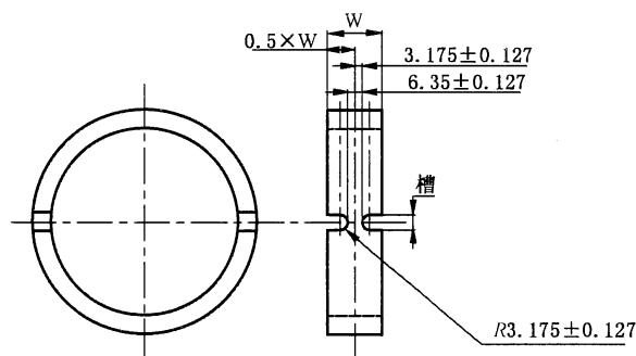
图 B.1 试样制作示意图
