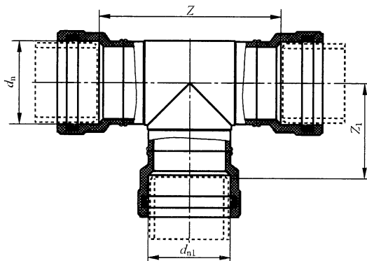
图 A.2 三承口三通示意图
