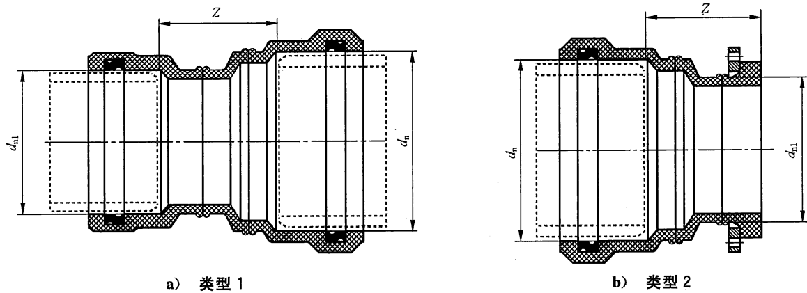
图 A.4 双承口变径和法兰承口变径示意图
