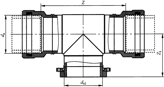
图 A.6 法兰支管双承口三通示意图
