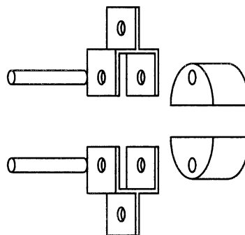
图 B.1 试样制作示意图
