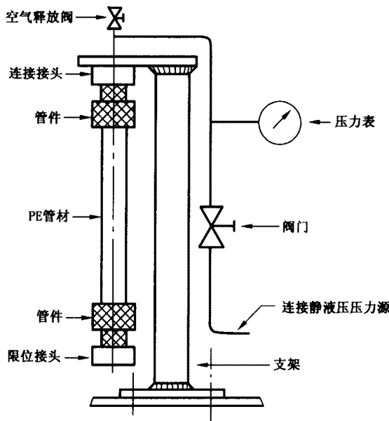
图 B.1 装置示意图
