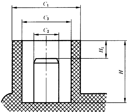
图 A.1 典型的 A 型接线端
