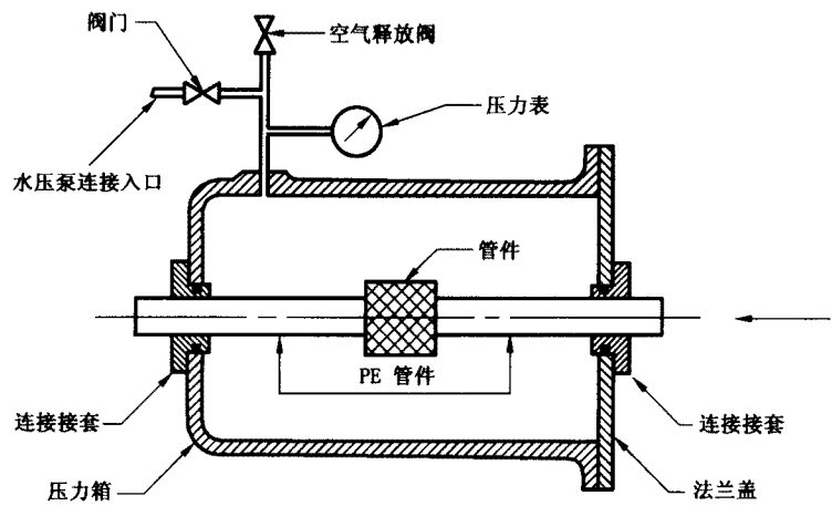
图 C.1 装置示意图
