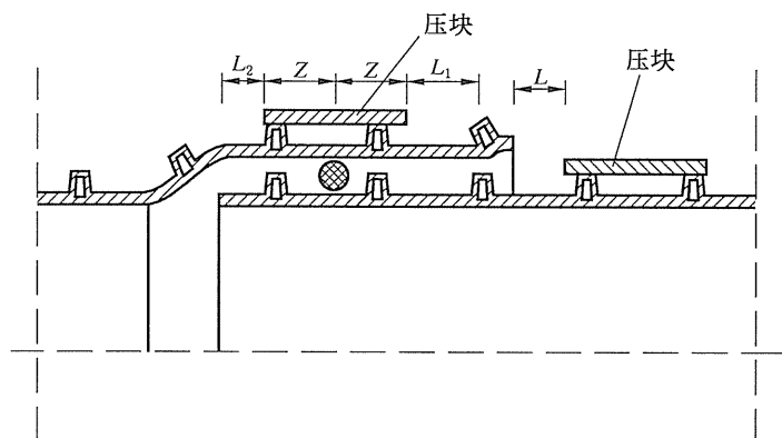
图 B.3 在连接密封处压块的定位
