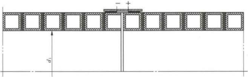
图 C.5 电热熔带连接示意图
