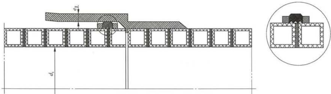
图 C.2 密封件位于插口的连接示意图
