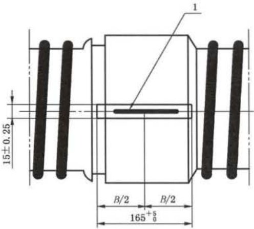
图 D.1 熔接处的拉伸力制备试样的位置和尺寸
