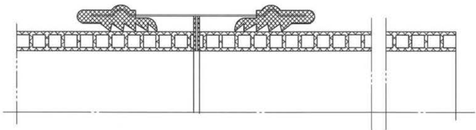
图 C.1 双向承插弹性密封连接示意图
