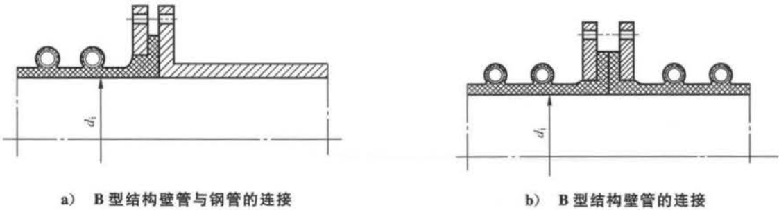
图 C.6 法兰连接示意图
