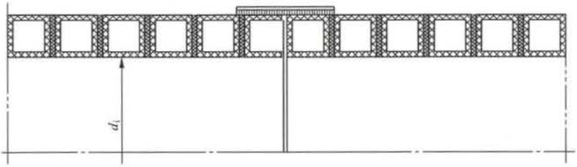
图 C.4 热收缩套连接示意图
