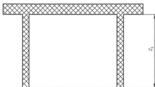
图 B.3 典型管堵示意图
