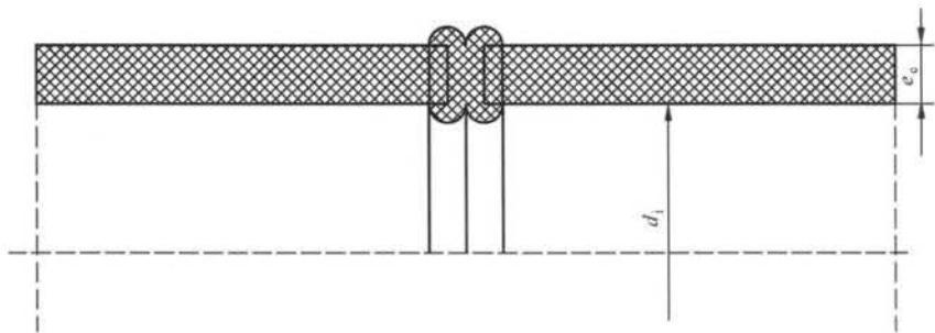
图 C.3 热熔对焊连接示意图
