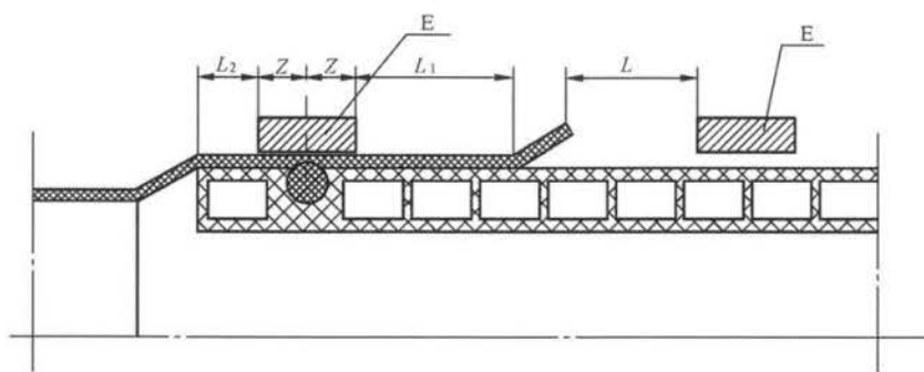
图 E.3 在连接密封处压块的定位
